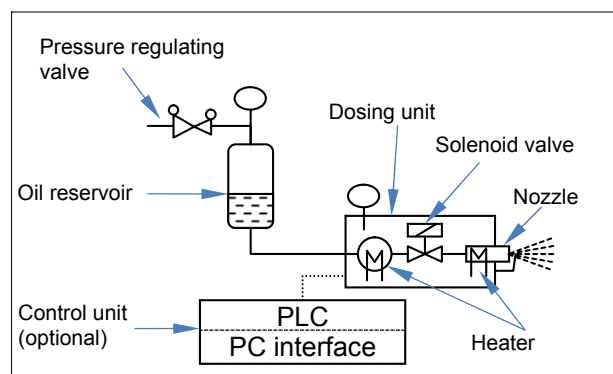
Funktional schematic
